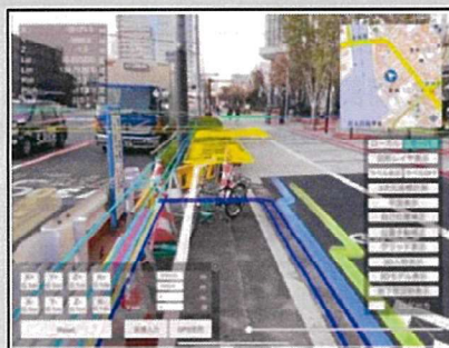
写真2 地下埋設物のAR表示
