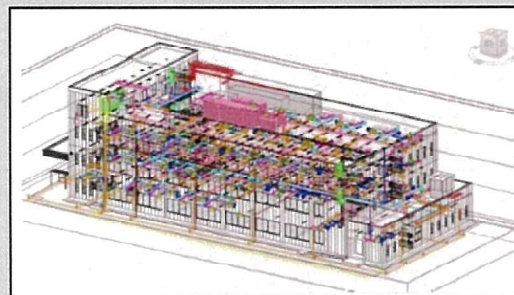
フルBIMモデル
