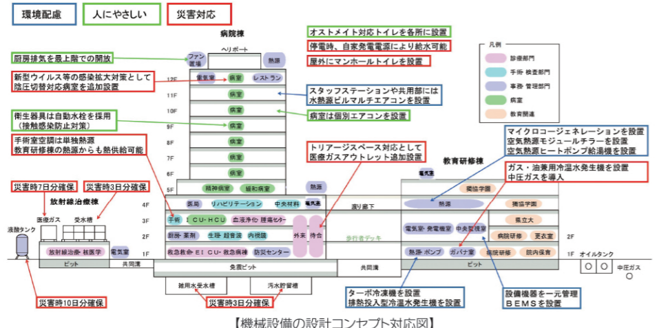
【機械設備の設計コンセプト対応図】
